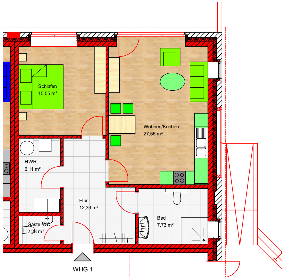
Grundriss WHG 1, rollstuhlgerecht 1:100
